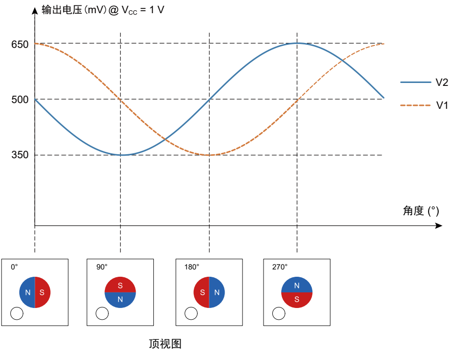
图 5-2 TMR3015F 输出信号与磁铁关系示意图
