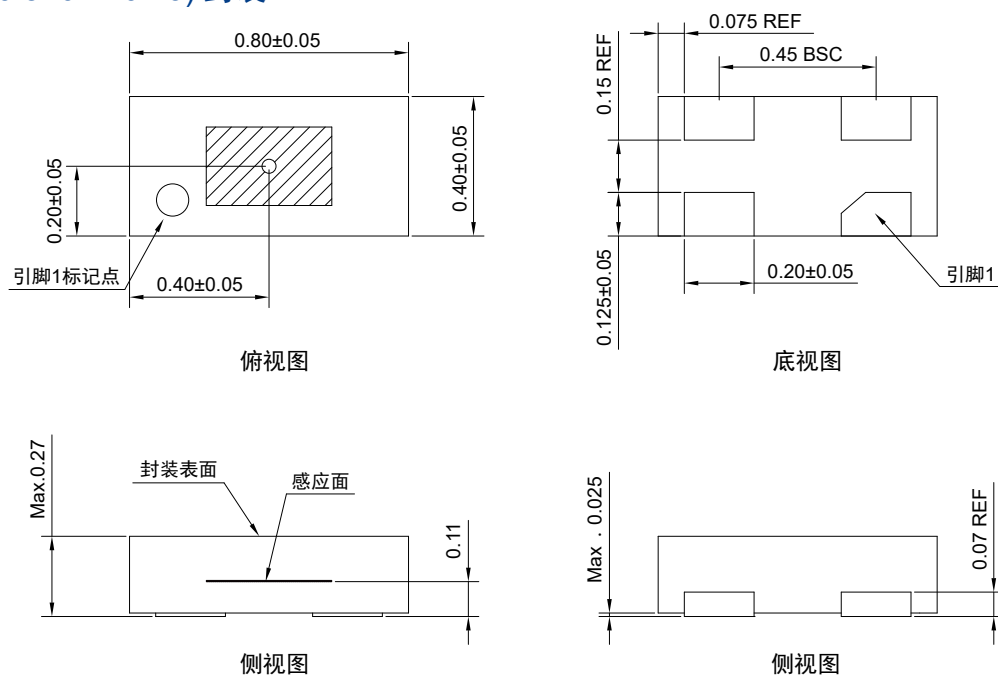
图 6 DFN4L(0.8×0.4×0.23) 封装图（尺寸单位：mm）
