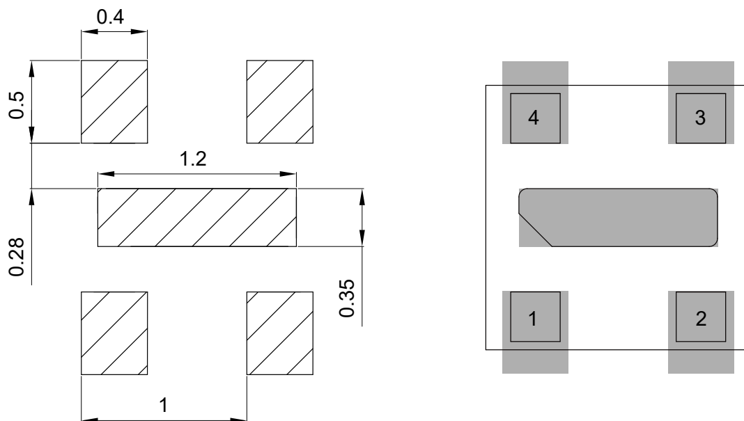
图 9 DFN4L(1.6×1.6×0.5) 焊盘尺寸推荐图 (尺寸单位: mm)
