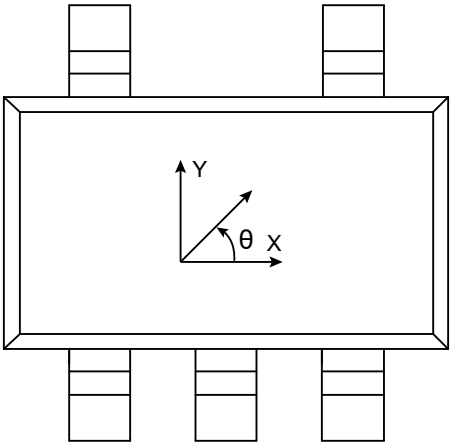
图 4-2 敏感方向（SOT23-5）
