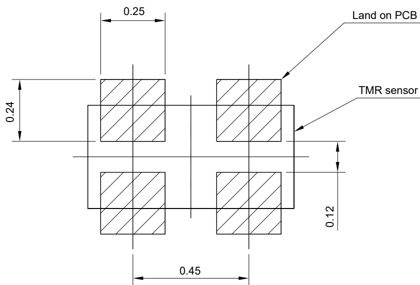
图 10 DFN4L(0.8×0.4×0.23) 焊盘尺寸推荐图 (尺寸单位: mm)
