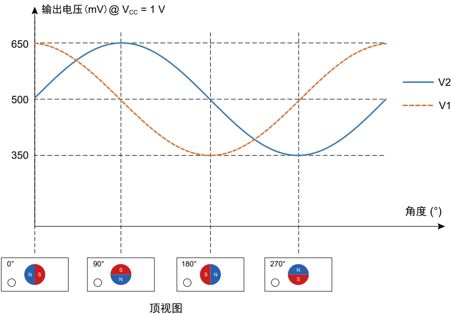
图 5-1 TMR3015D 输出信号与磁铁关系示意图
