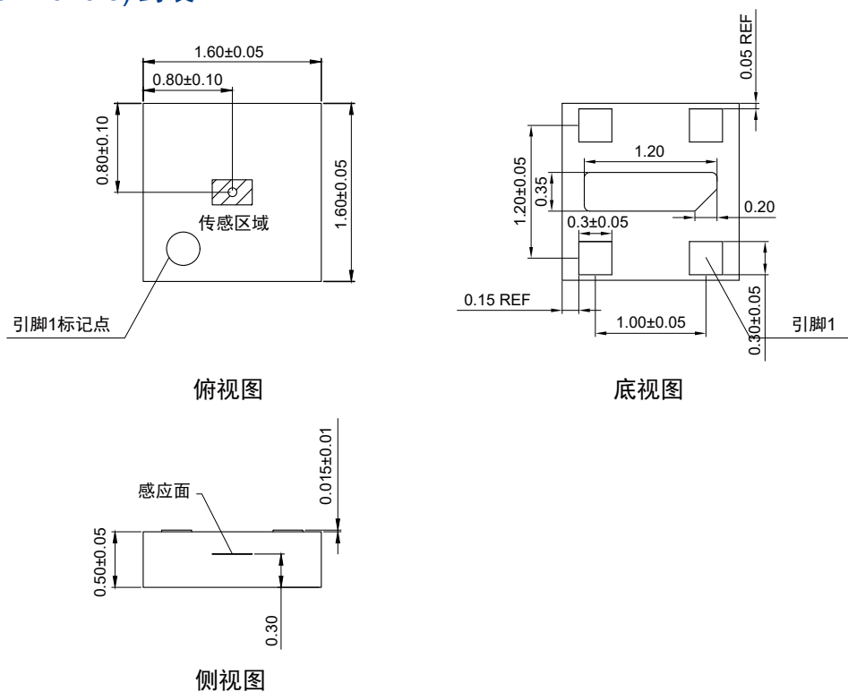
图 7 DFN4L(1.6×1.6×0.5) 封装图（尺寸单位：mm）
