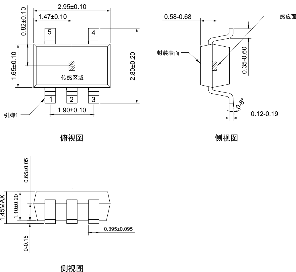
图 8 SOT23-5 封装图（尺寸单位：mm）
