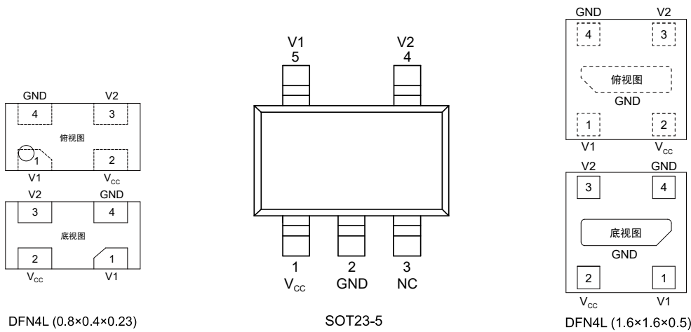
图 2 引脚定义
