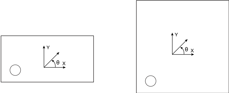
图 4-1 敏感方向（DFN4L）
