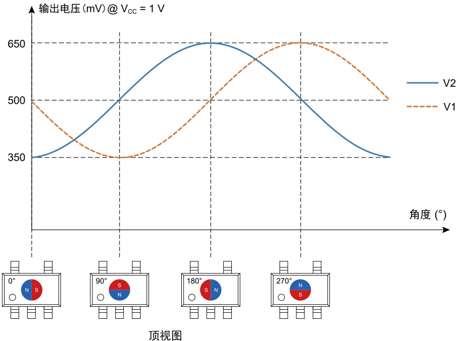
图 5-3 TMR3015S 输出信号与磁铁关系示意图
