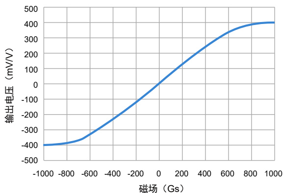
TMR2084 ±1000 Gs 输出曲线
