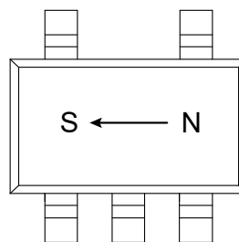
图 2 芯片敏感方向 (SOT23-5)
