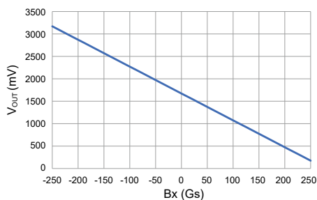
图 3 TMR2625D-AAI 芯片 X 轴输出曲线
