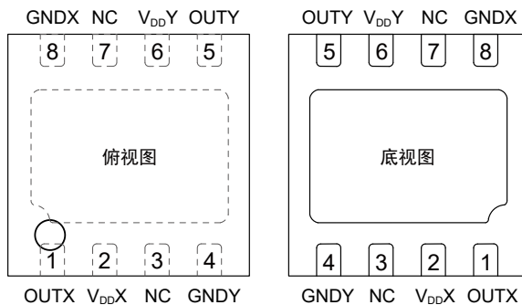
图 5 引脚定义 (DFN8L)
