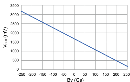
图 4 TMR2625D-AAI 芯片 Y 轴输出曲线
