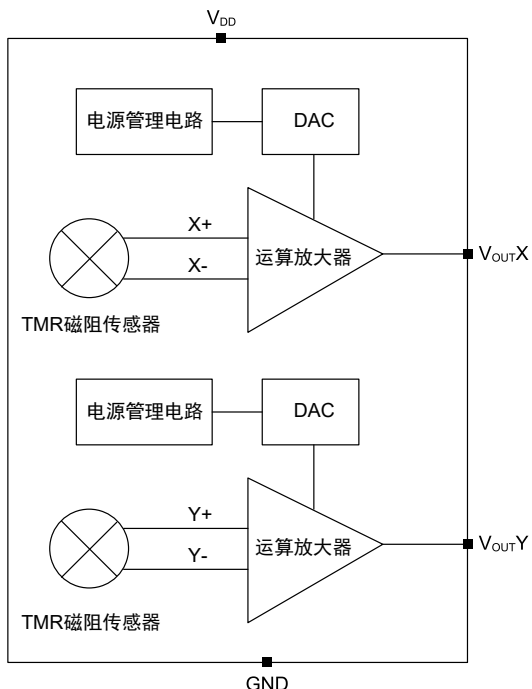
图 1 芯片内部原理框图
