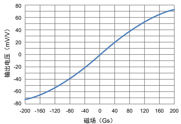
TMR2585 ±200 Gs 输出曲线
