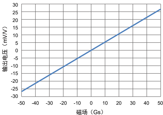
TMR2585 ±50 Gs 输出曲线
