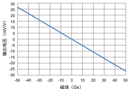
图 2 TMR2585 芯片输出曲线
