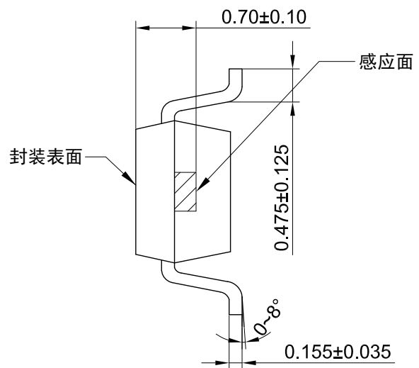
侧视图
