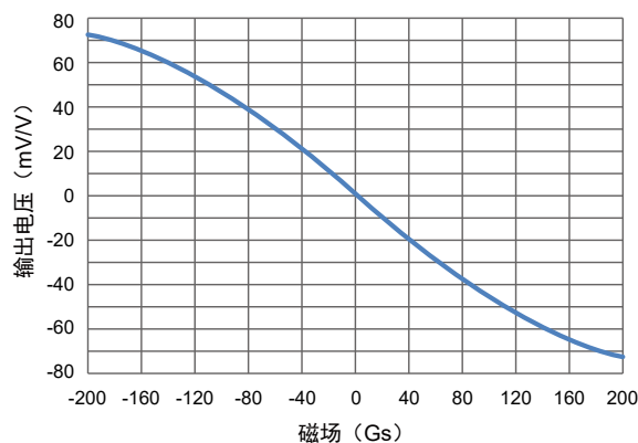
TMR2585 ±200 Gs 输出曲线
