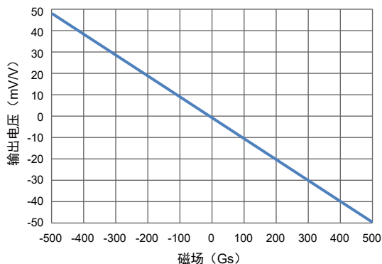
图 2 TMR2583 芯片输出曲线
