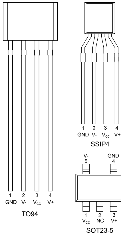
图 3 引脚定义
