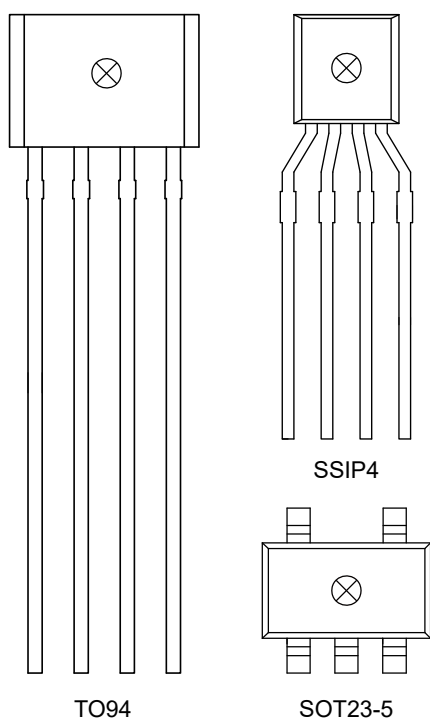
图 1-2 芯片轴向图（俯视图）
