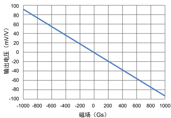
TMR2583 ±1000 Gs 输出曲线
