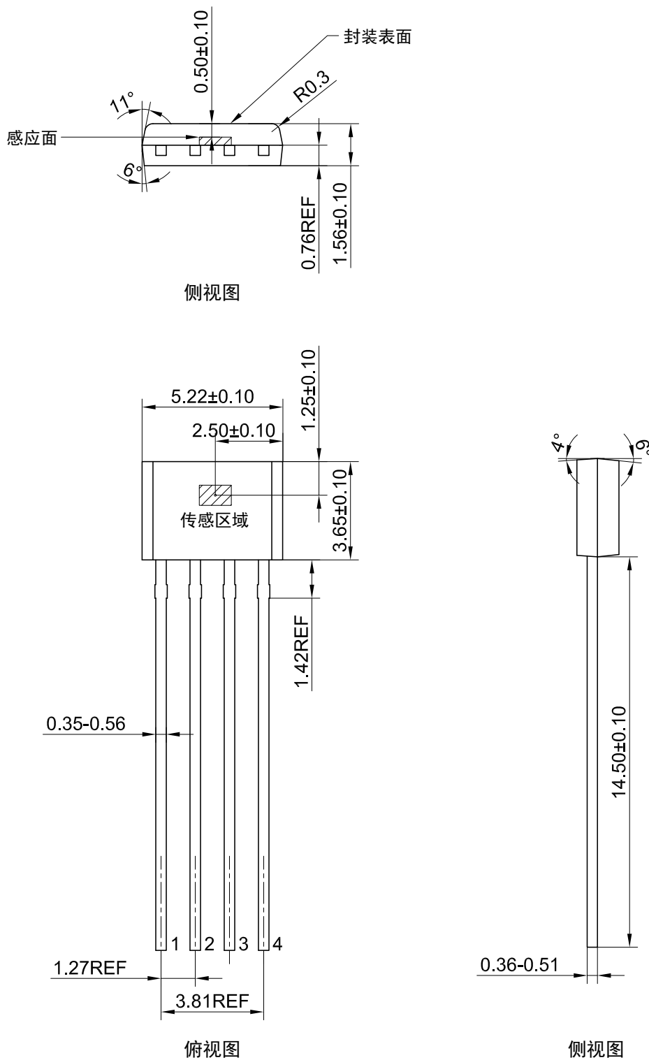
图 4 TO94 封装图 (尺寸单位: mm)
