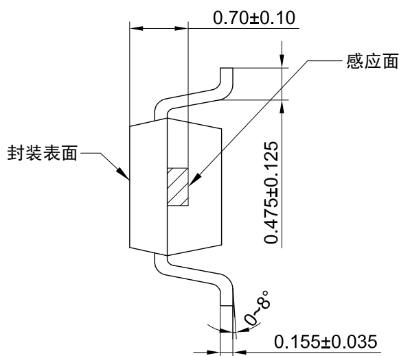
侧视图
