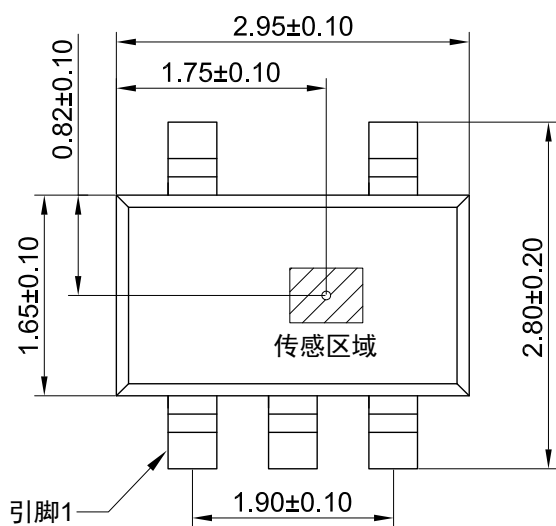
俯视图
