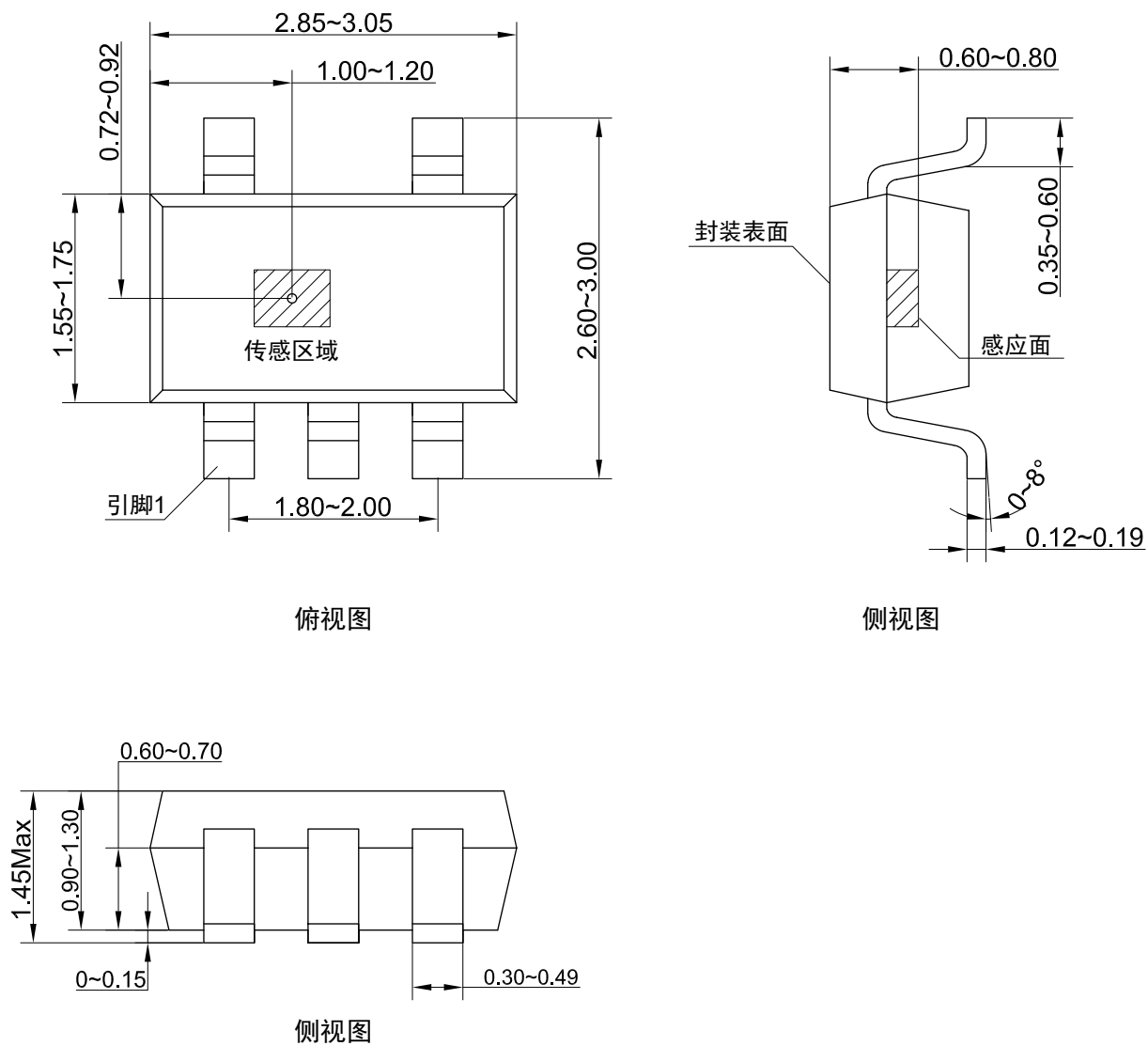
图 3 SOT23-5 封装图 (尺寸单位: mm)
