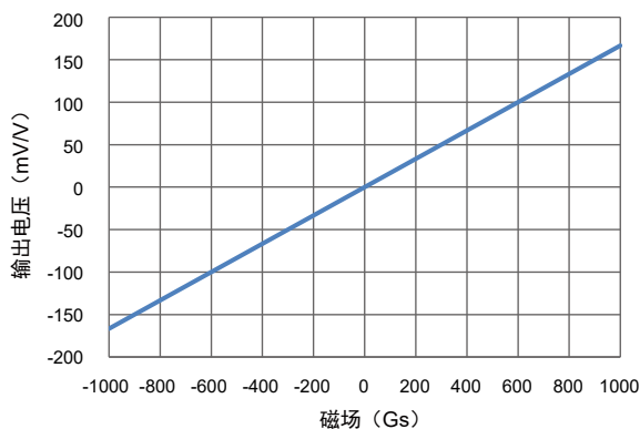
TMR2083 \pm 1000 Gs 输出曲线
