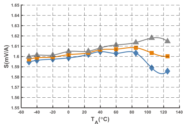
图 17 灵敏度曲线 (@ I_{PN} = 2500\text{ A} )
