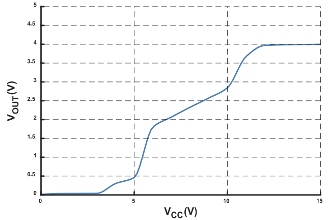
图 2 输出特性与供电电压曲线 (@I P = I PN )
