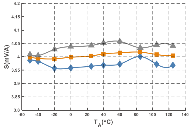
图 13 灵敏度曲线 (@ I_{PN} = 1000\text{ A} )
