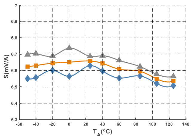
图11 灵敏度曲线 (@I PN = 600 A)
