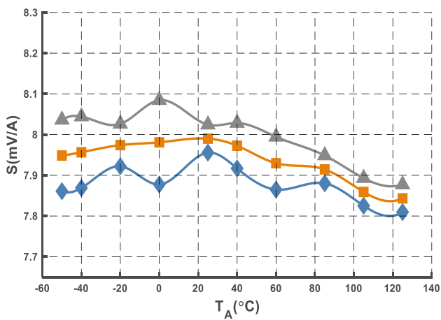
图10 灵敏度曲线 (@I PN = 500 A)
