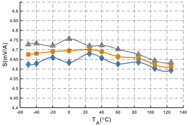
图 12 灵敏度曲线 (@ I_{PN} = 850\text{ A} )
