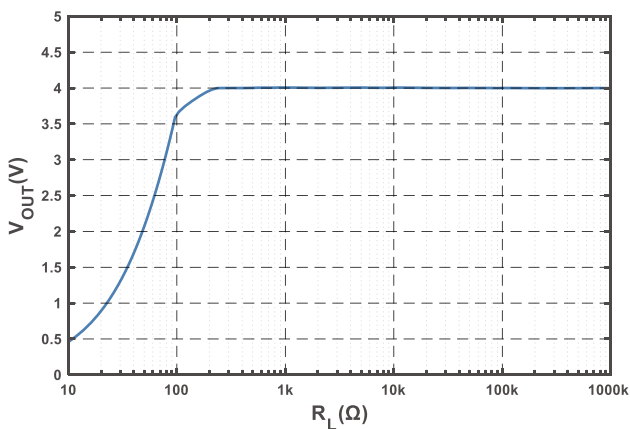
图 3 负载电阻特性曲线 (@I P = I PN )
