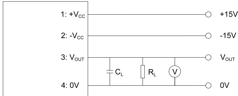
图 21 电气接口接线图
