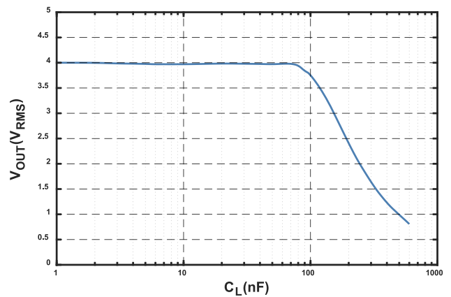
图 4 负载电容特性曲线 (@I P = I PN )
