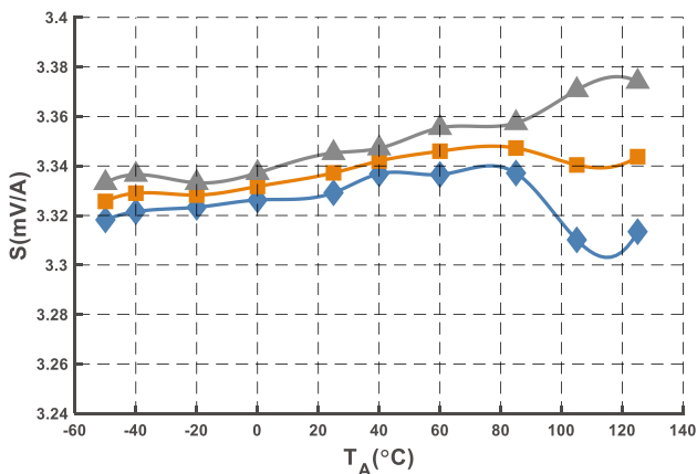
图 14 灵敏度曲线 (@ I_{PN} = 1200\text{ A} )
