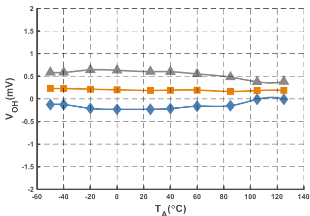
图 19 磁滞特性曲线
