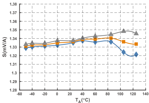
图 18 灵敏度曲线 (@ I_{PN} = 3000 A)
