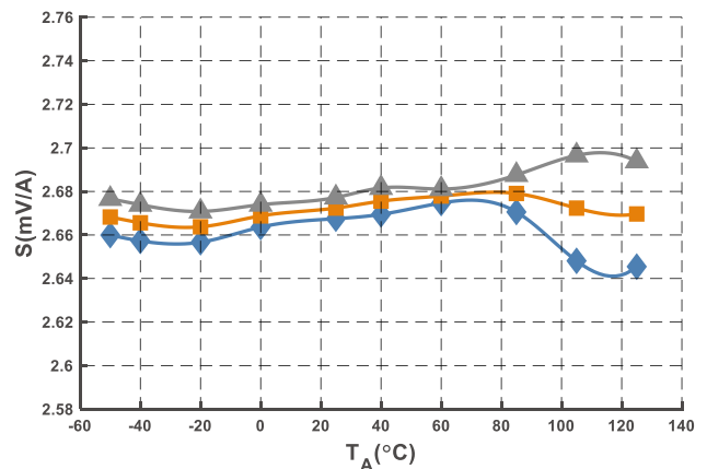
图 15 灵敏度曲线 (@ I_{PN} = 1500\text{ A} )
