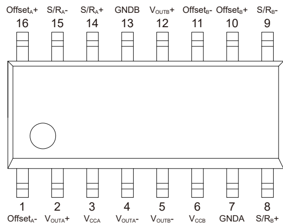
图 4 引脚定义
