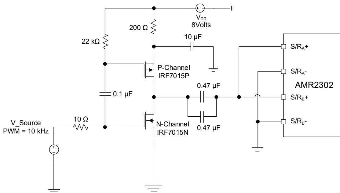
图 8 AMR2302 应用电路图
