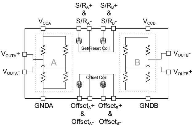
图 1 芯片内部原理框图
