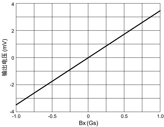
图 3-2 AMR2302 芯片输出曲线 (B 轴)
