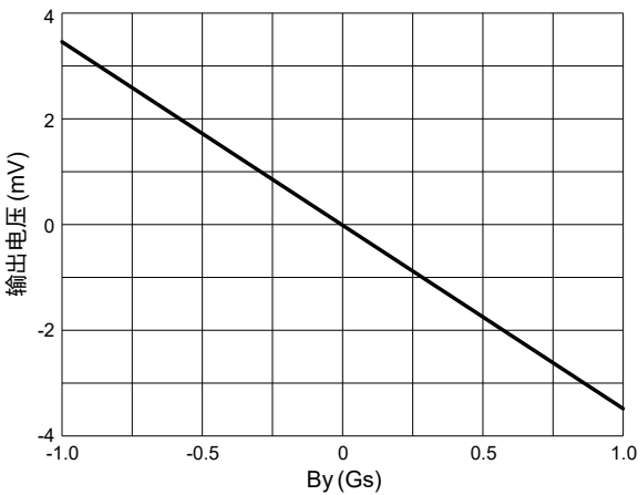
图 3-1 AMR2302 芯片输出曲线 (A 轴)
